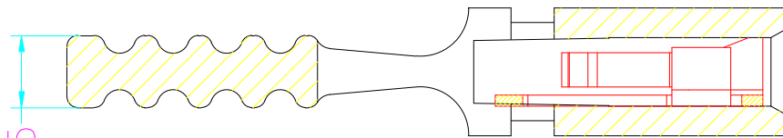
SECTION A-A
